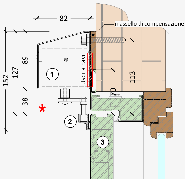
External flush door
