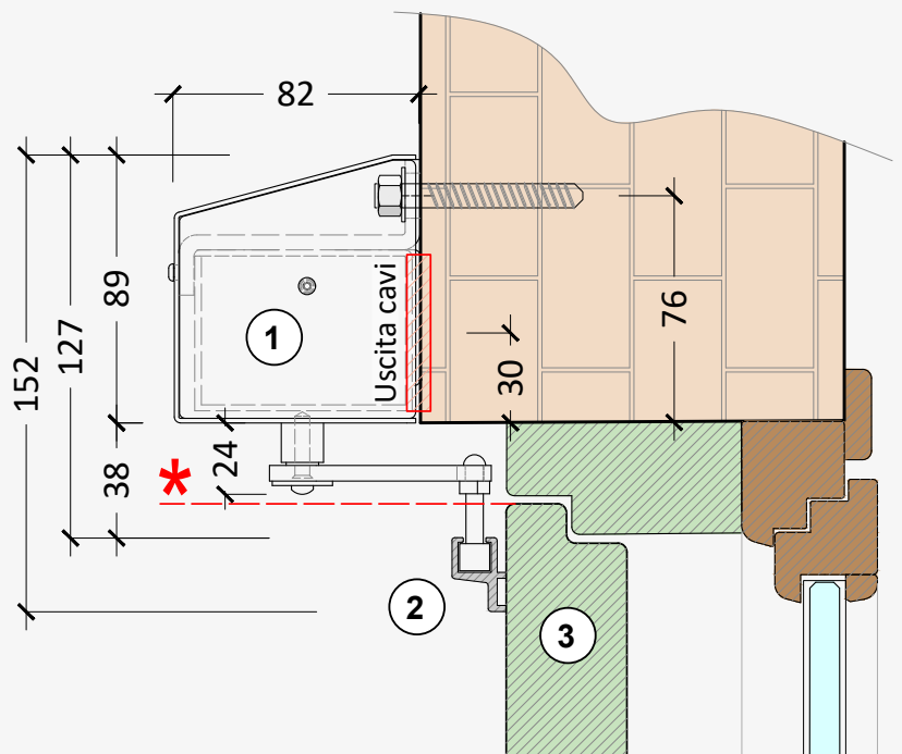
Anta con battuta in mazzetta
