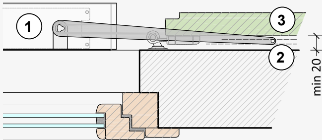
Bandella dritta cardine a murare
