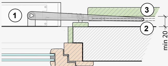
Bandella dritta e spalletta rivestita
