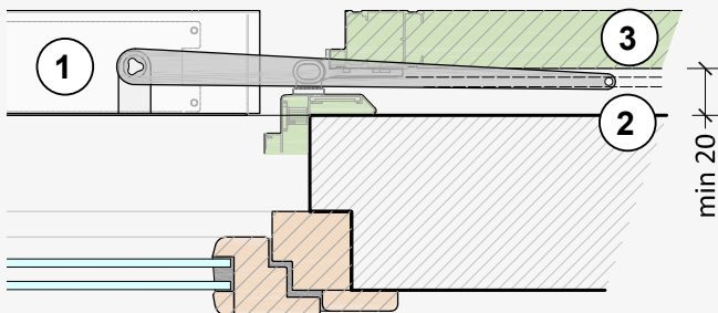
Bandella dritta e cardine su telaio in alluminio
