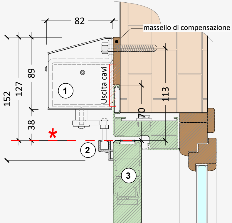
Anta a filo muro esterno
