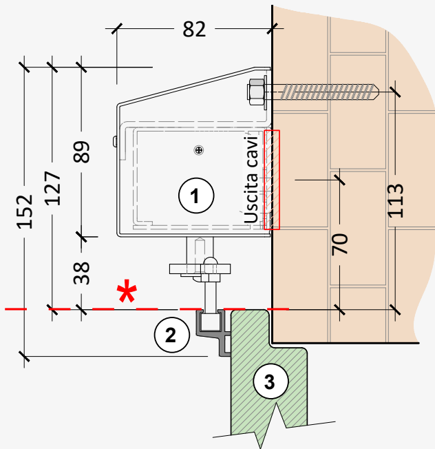
Anta tradizionale con battuta
